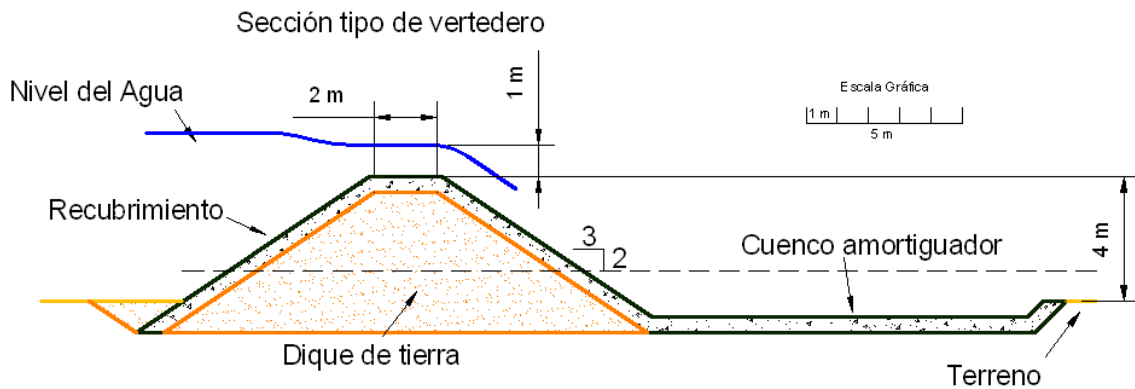
Figura 15.- Posible sección tipo de los vertederos del dique distribuidor. El dique mismo tendría obviamente al menos 1m más de altura.
