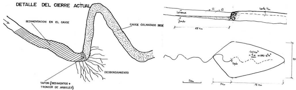
Figura 4.- Croquis de un tapón del río en planta (izquierda) y en perfil longitudinal (arriba, derecha) y esquema del área de derrame y sedimentación (derecha, abajo).
