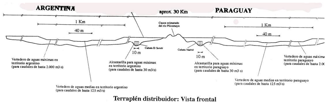
Figura 14.- Croquis del perfil longitudinal típico del dique de 1995 [11]
