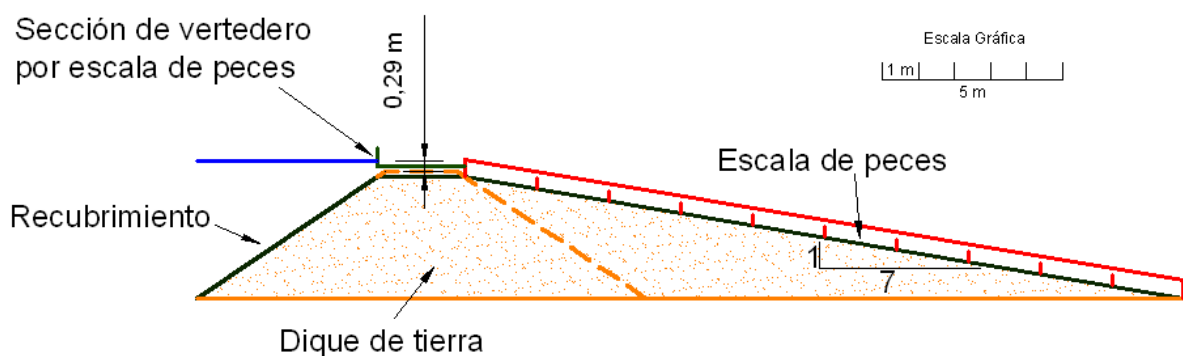
Figura 16.- Posible sección tipo de las escalas de peces que ocuparían el lugar central del dique distribuidor.
