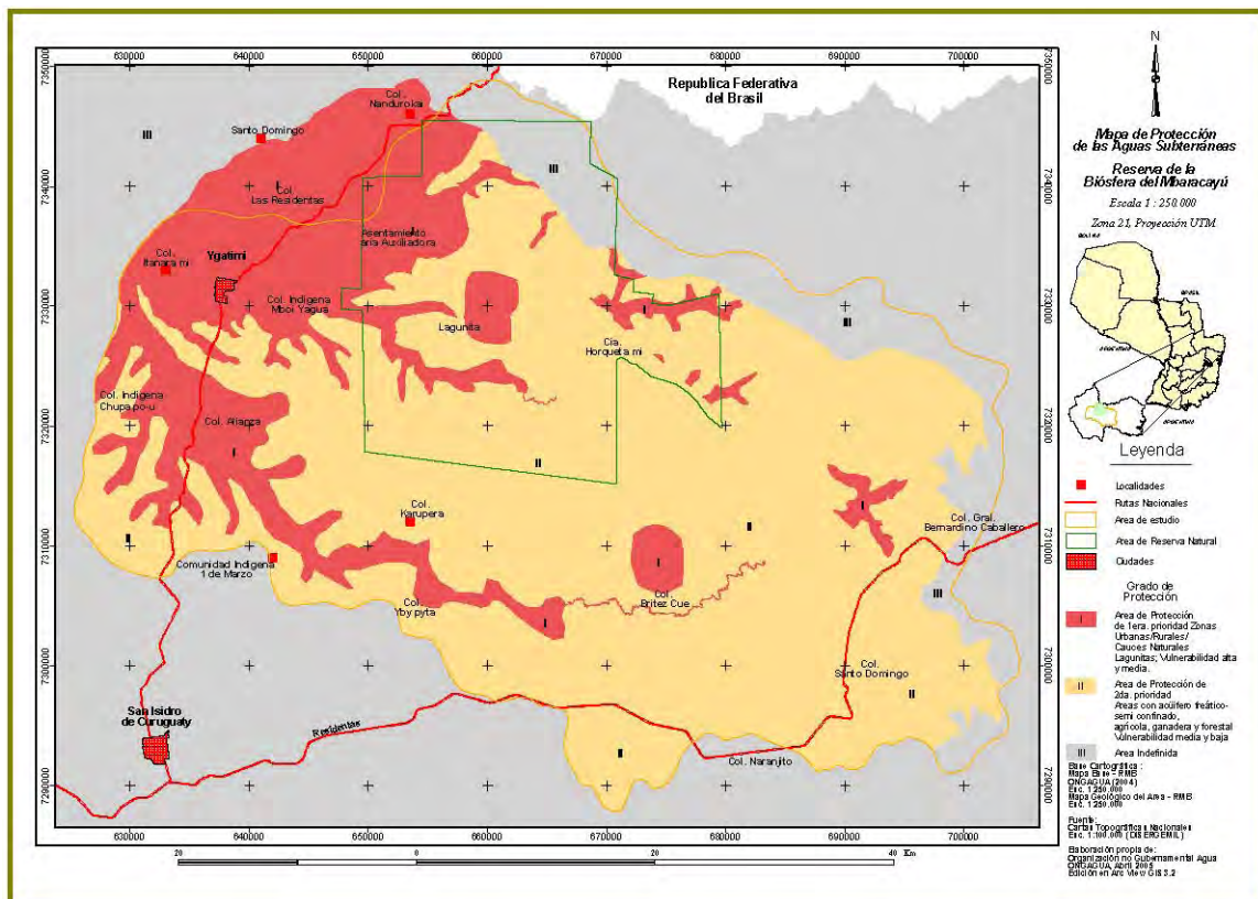
Figura 9. Mapa de Riesgo a la Contaminación del Agua Subterránea del área de Biosfera de la Reserva del Bosque Mbaracayá.
