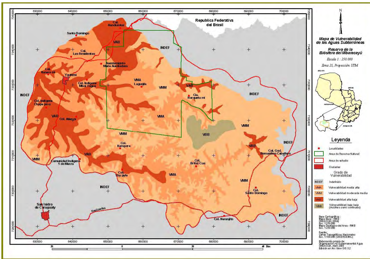
Figura 7. Mapa de vulnerabilidad del acuífero freático y semi-confinado de la Reserva del Bosque Mbaracayú
